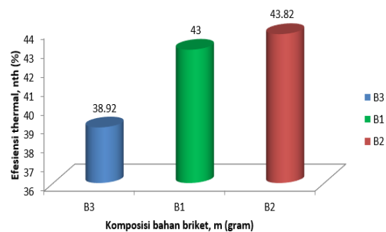
Gambar 5. Efisiensi thermal
