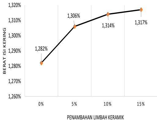
Gambar 4.3 Grafik Hubungan antara Penambahan Limbah Keramik dengan Berat Isi Kering Hasil Pemadatan
